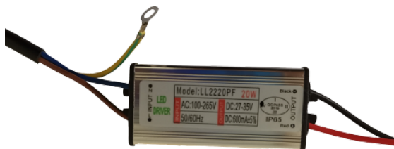
Драйвер для светодиодных светильников Led Favourite LL2220PF 600mA 20W IP65
