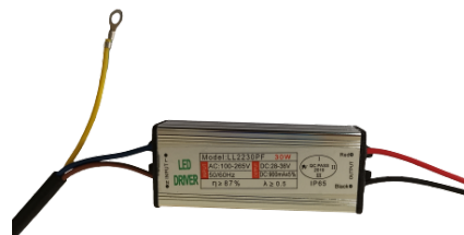
Драйвер для светодиодных светильников Led Favourite LL2230PF 900mA 30W IP65
