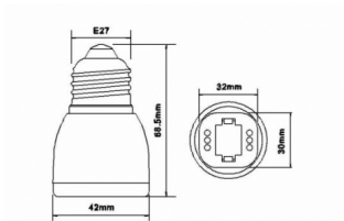
Адаптер PBT 1S220 g23 -e27
