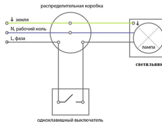
Схема установки светильника 220В
