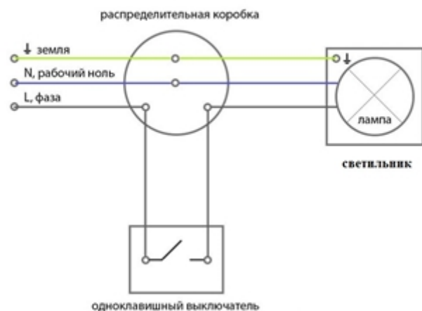
Схема установки светильника 220В
